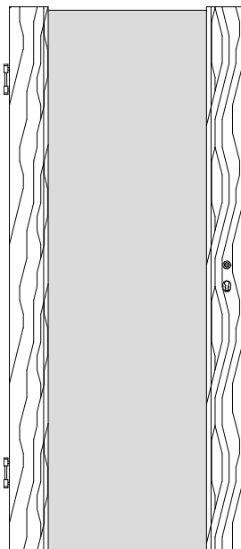
LE/HG mit 8 mm ESG
